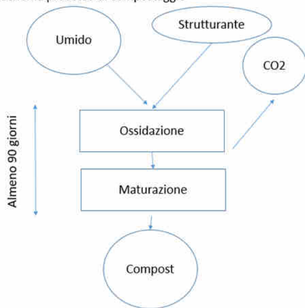
Schema processo di compostaggio
