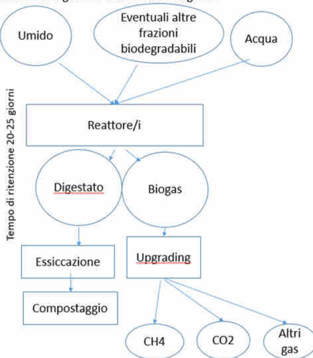
Schema di digestore anaerobico integrato
